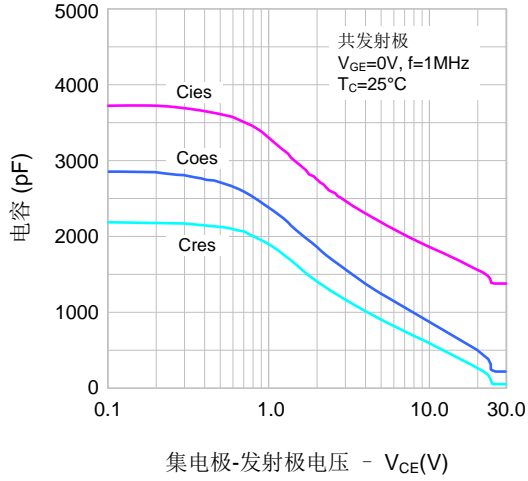
图7. 电容特性
