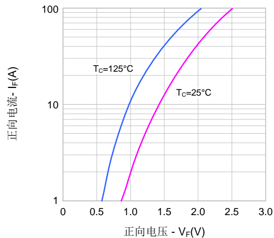
图12. 正向特性
