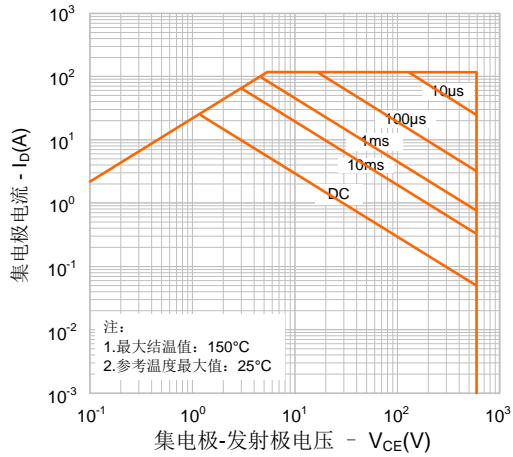
图15. 最大安全工作区域
