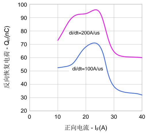
图 14. 反向恢复电荷VS.正向电流
