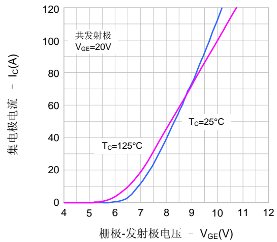
图4. 传输特性
